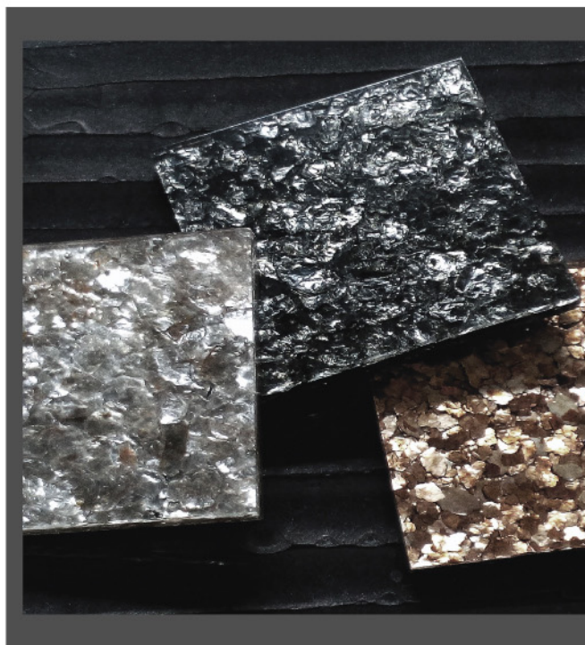
白雲母
